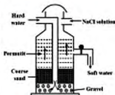
Fig: 10.6 Permutit method
