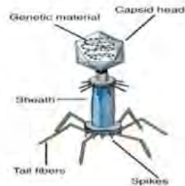
Fig. 3.24 bacteria
