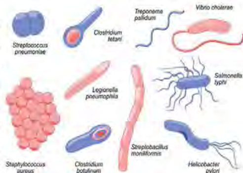
Fig. 3.25 bacteria
