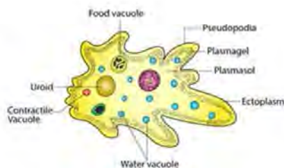
Fig. 3.26 Amoeba
