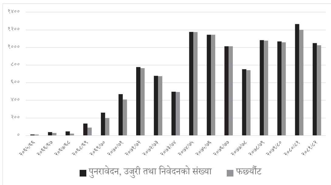
चार्ट नं. १ : पुनरावेदनको अवस्था
