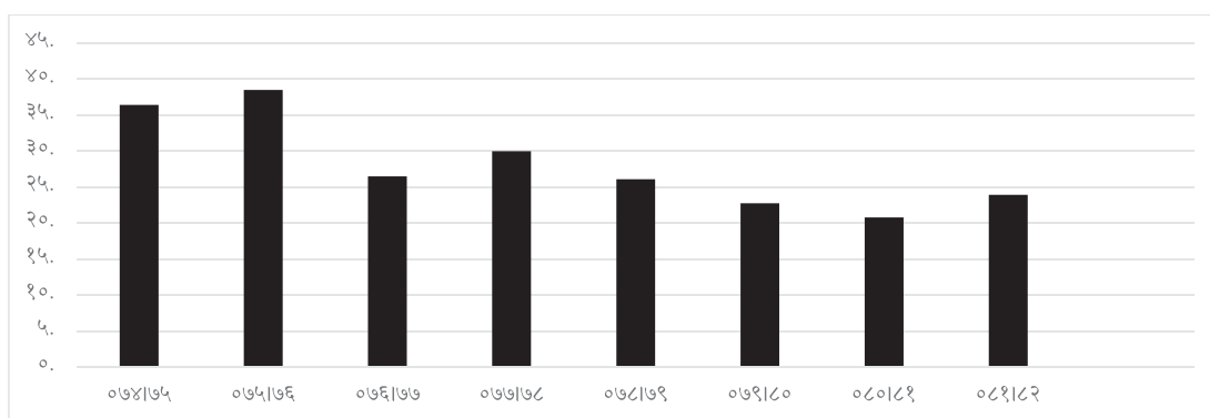
चार्ट नं. ४ : कार्यक्रममा विनियोजन भएको बजेटको प्रतिशत
