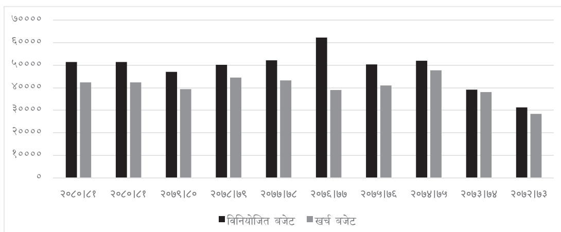
चार्ट नं. २ : विगत दश वर्षको विनियोजित बजेट र खर्चको विवरण
