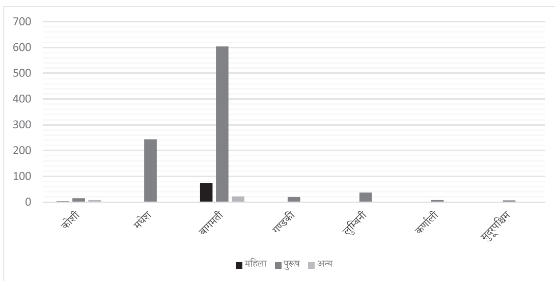
चार्ट नं. १ : प्रदेशगत पुनरावेदनको अवस्था
