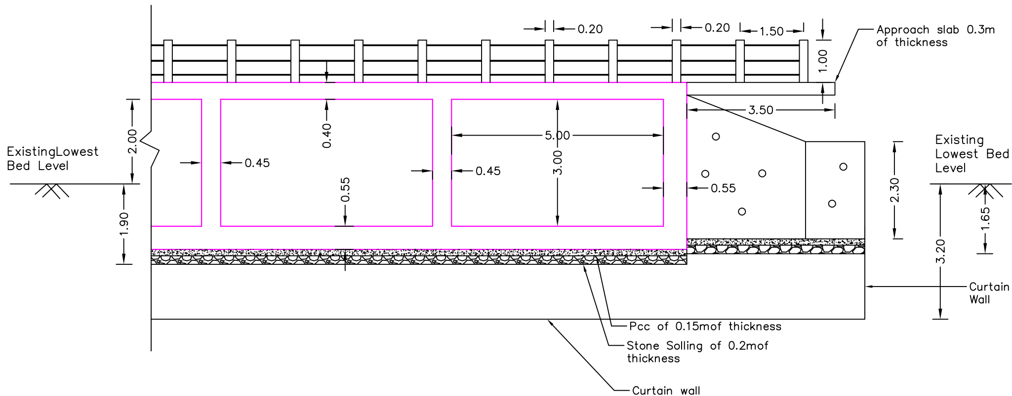
Fig: B-B section
